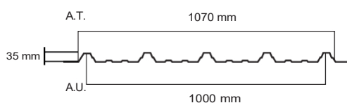
DIMENSIONES DE PANEL TERMOACÚSTICO MULTICAPA KLAR TK5 PRO
