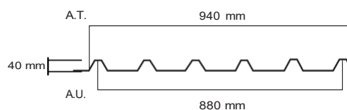
DIMENSIONES DE PANEL TERMOACÚSTICO MULTICAPA KLAR TK6S PRO
