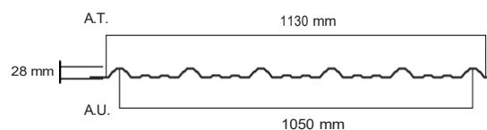
DIMENSIONES DE PANEL TERMOACÚSTICO MULTICAPA KLAR TK6 PRO
